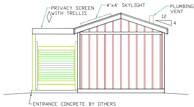
RIGHT ELEV.
